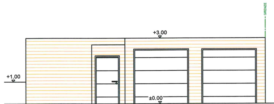
Ansicht Süd
